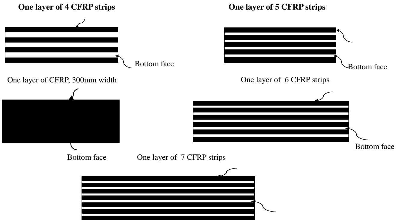
Fig. (6): CFRP Details
